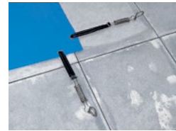
STAR: Gurt + Dynamometerfedern & Kunststoffösen
